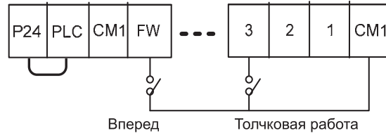
Рис. 9-13 Выбор толчкового функционирования в программируемой входной клемме
