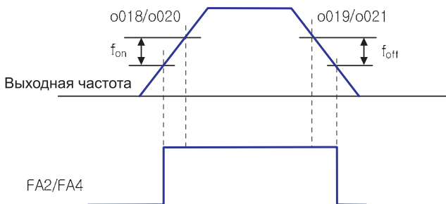
Рис10-9 Вывод чрезмерно установленной частоты (2 : FA2, 19 : FA4)
