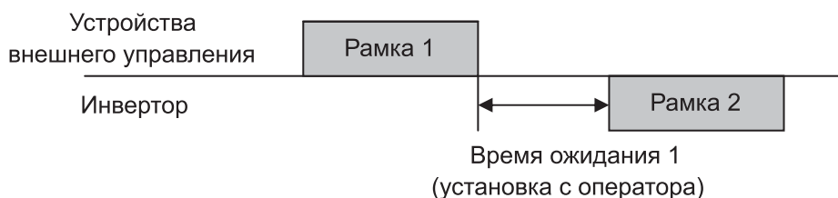
Рис. 13-3 Порядок связи
