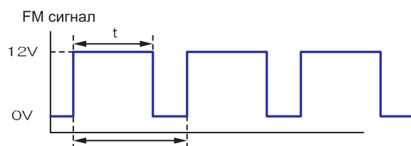
Рис. 10-12 Временная диаграмма FM сигнала (o009 = 0, 1, 2, 4, 5, 6, 7)
