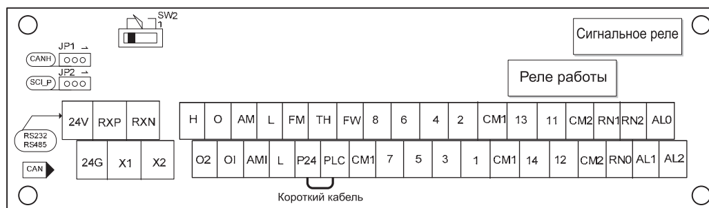
Рис. 9-1 Компоновка клемм цепи управления
