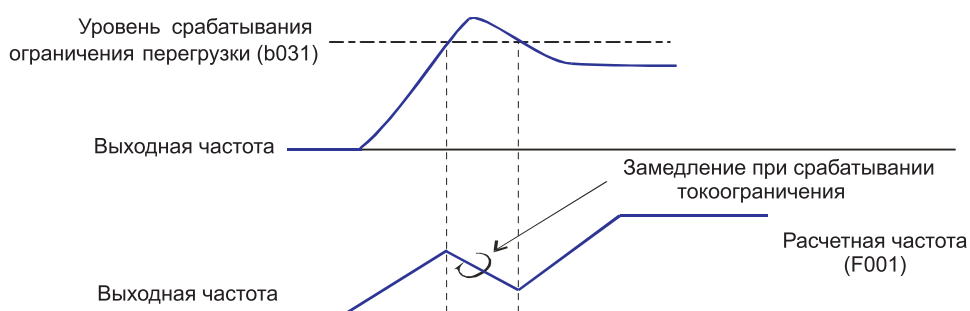
Рис. 8-10 Временная диаграмма предварительного извещения токоограничения (b030~b033)
