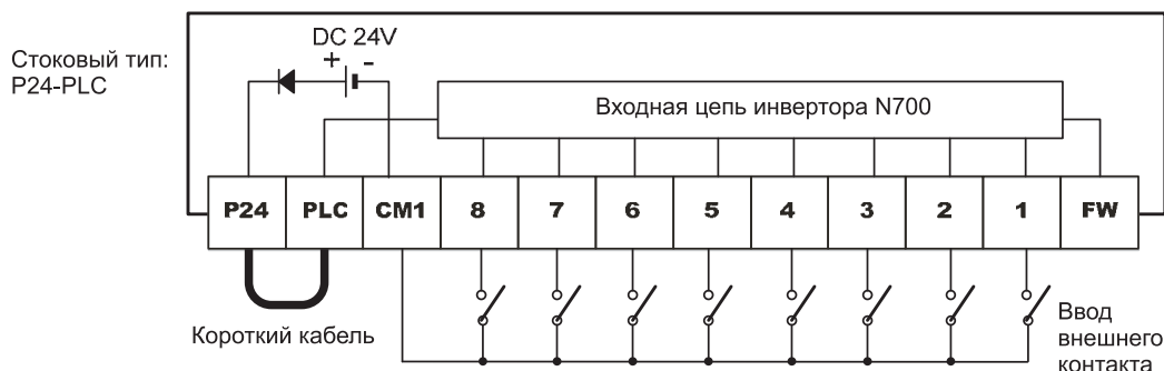
Рис. 9-3 Соединение микропроцессорной входной клеммы (Стоковый тип: P24-PLC)
