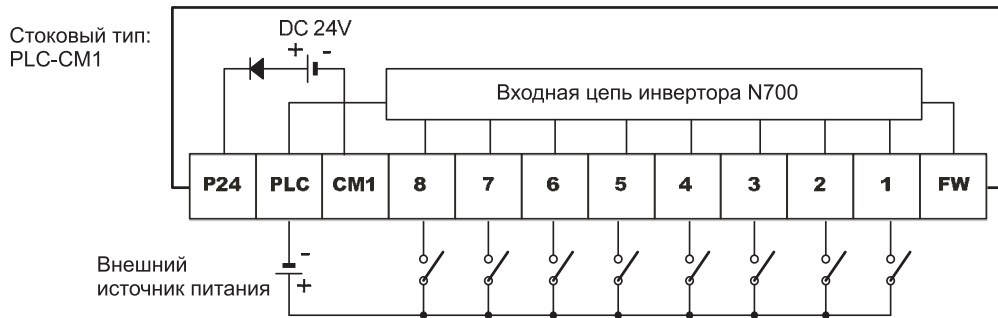
Рис. 9-5 Соединение микропроцессорной входной клеммы (Тип источника: PLC-CM1)
