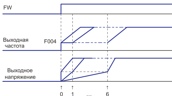
Рис. 8-1 Кривая выбора пуска со сниженным напряжением
