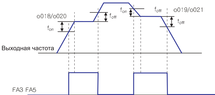
Рис. 10-10 Установка частоты вывода (6 : FA 3, 20 : FA 5)
