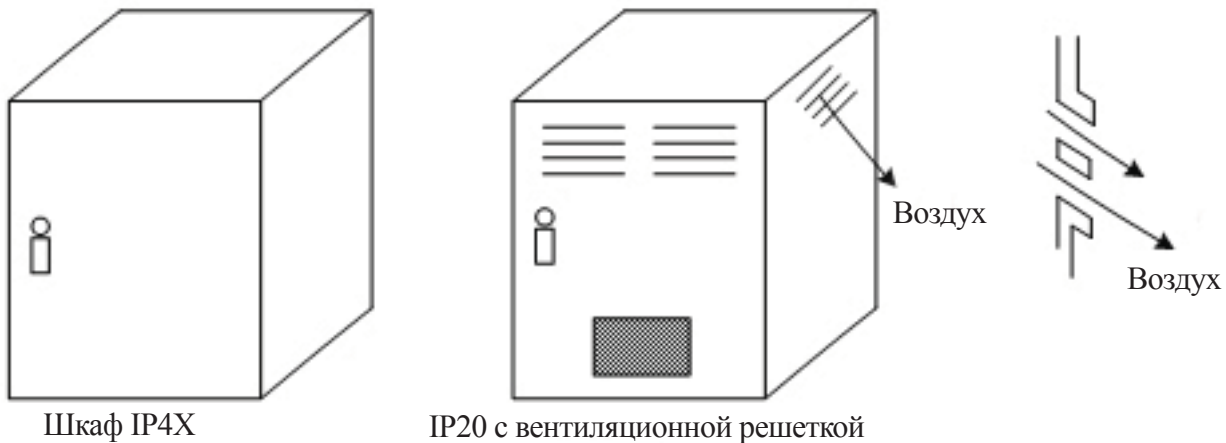
Рис. 1 Шкаф инвертора
