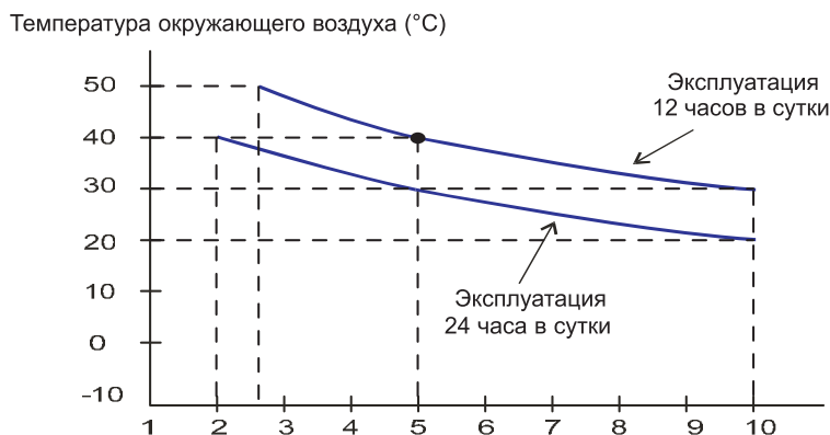
Рис. 15-1 Срок службы
