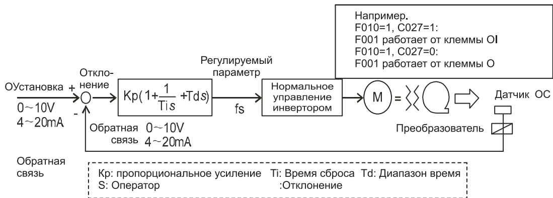
Рис. 11-6 Базовая блок-схема ПИД управления
