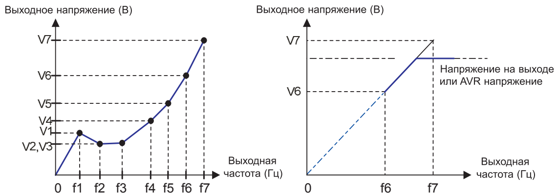
Рис. 7-5 Кривая произвольной установки V/f
