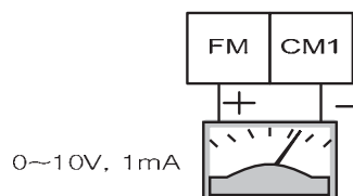
Рис. 10-13 Метод отображения FM сигнала с использованием аналога
