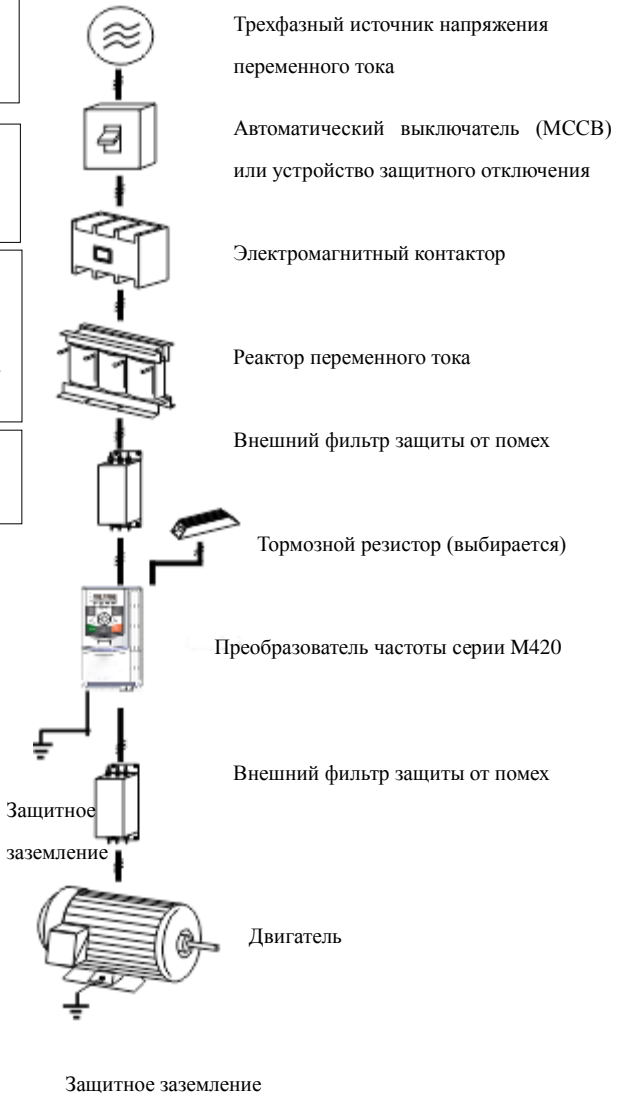
Рис. 1. Иллюстрация подключения периферийных устройств
