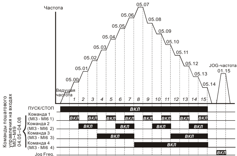
Пошаговое управление скоростью через внешние терминалы
