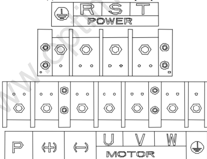
Рис. 2-17 Силовые клеммы приборов 200-400 кВт
