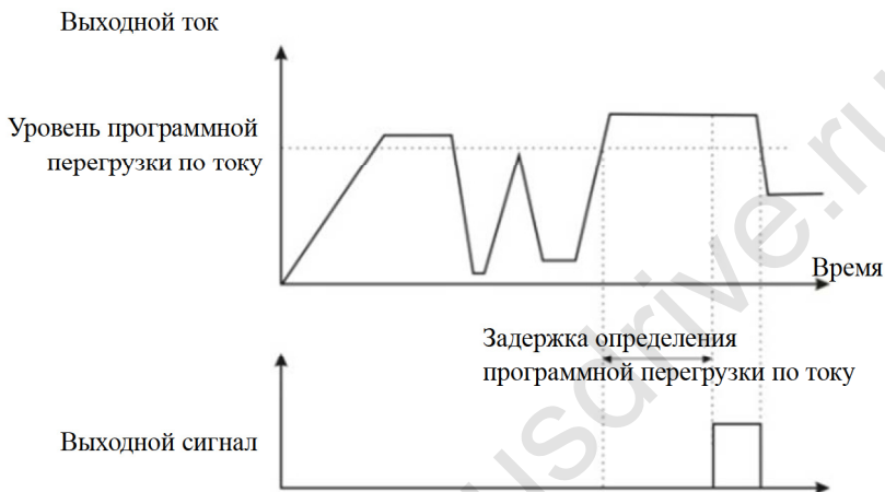
Рис. 6-19 Программное определение перегрузки по току
