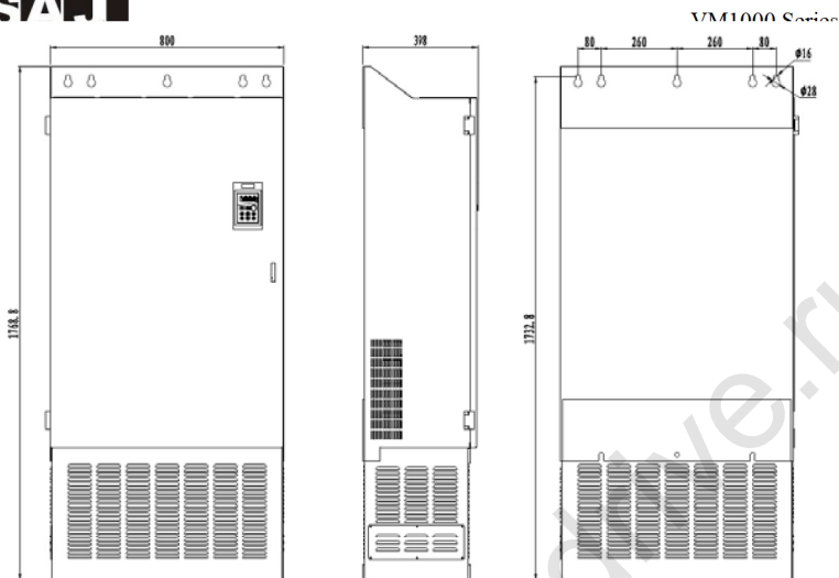
Рис. 1-8 Габариты и монтажные размеры ПЧ 200-280 кВт
