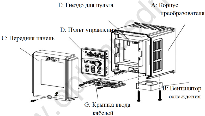
Рис. 2-1 Конструкция преобразователя (0,75...7,5 кВт, 11 кВт тип Р)
