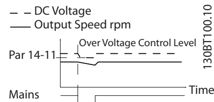
Рисунок 3.39 Кинетический резерв, короткое замыкание сети. Скачок длится, пока в системе есть энергия.
