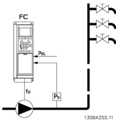
Рисунок 3.51 Условные обозначения: FC=преобразователь частоты; fo=частотный выход; Ps=P системы; PsL=P задан.
