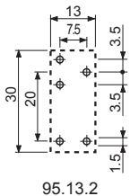
Вид со стороны выводов
