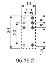
Вид со стороны выводов
