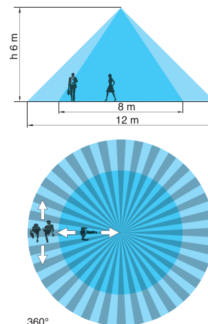
18.31...0031 - Монтаж в помещениях с высокими потолками
