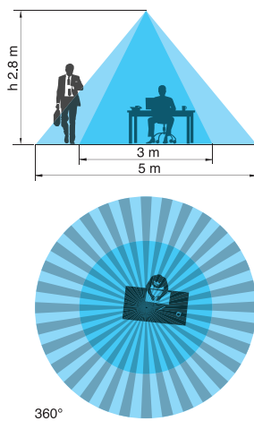
18.31...0031 - Монтаж на поверхности на потолке в помещении
