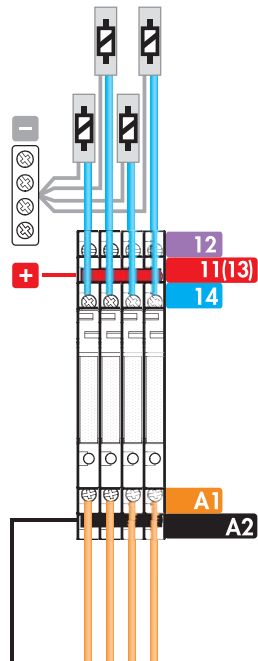
Выход PLC
